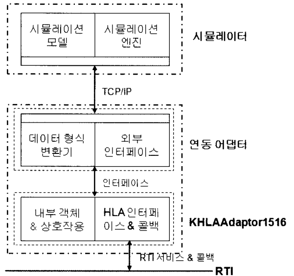
[그림 3] HLA/RTI 연동 어댑터 구조
