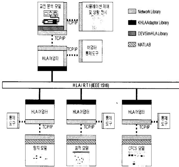
[그림 11] HLA 아댑터를 이용한 연동 시뮬레이션
