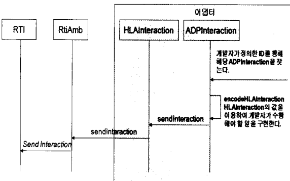
[그림 9] 상호작용 전송(Send Interaction)
