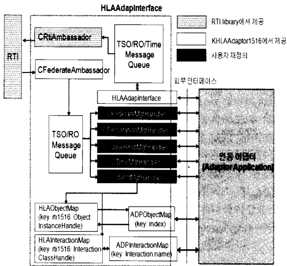
[그림 6] KHLAAdaptor1516 전체 구조 [4,9]
