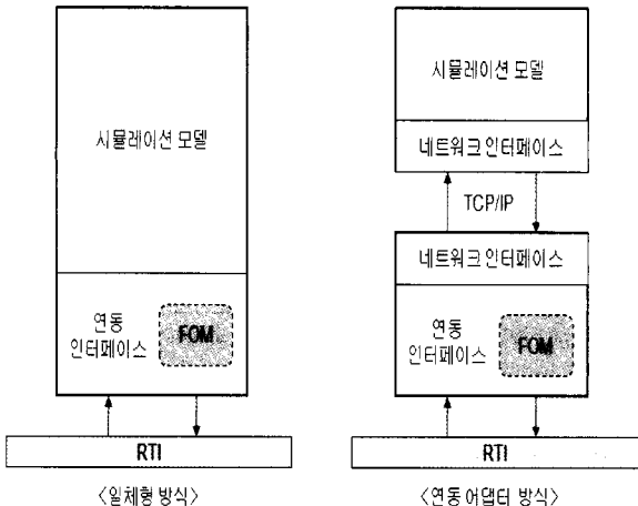
[그림 2] 데이터 형식 변환의 위치에 따른 연동 인터페이스 방식의 비교
