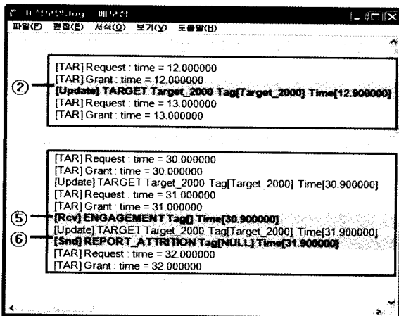
(d) 표적모델의 이벤트로그
