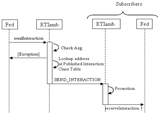
그림 6. sendInteractionWithRegion() 서비스
