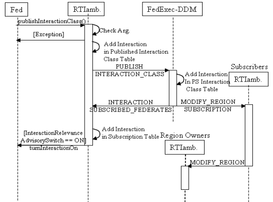
그림 5. publishInteractionClass() 서비스
