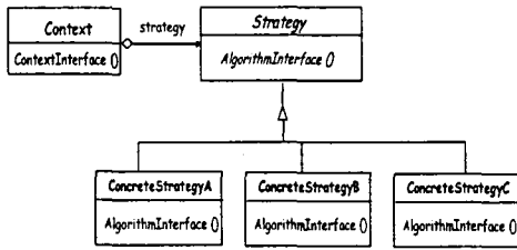
그림 1 Strategy 패턴
